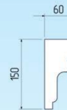
Молдинг 024 150 мм x 60 мм ПП - 4 мм
