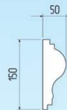
Молдинг 023 150 мм x 50 мм ПП - 4 мм
