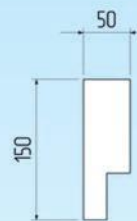
Молдинг 022 150 мм x 50 мм ПП - 4 мм
