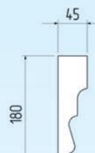
Молдинг 028 180 мм x 45 мм ПП - 4 мм
